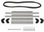
iM2300-M4-BEZEL-L Lunette du couvercle (métrique)
